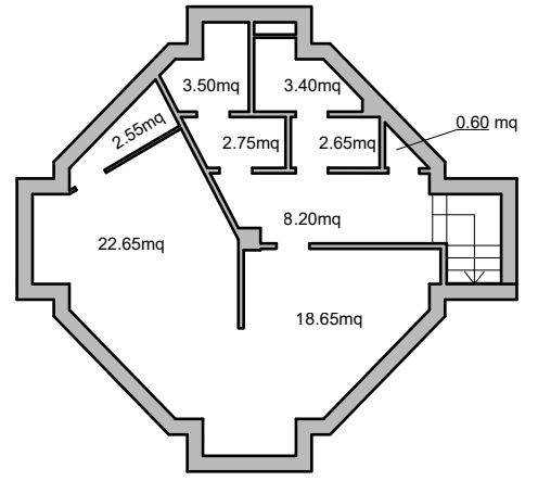
PIANO PRIMO SOTTERRANEO
