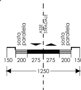
Tipologie sezioni stradali – strada locali in ambito urbano - (Fig. 3.6.i del D.M. n°6792 del 05/11/2001)
